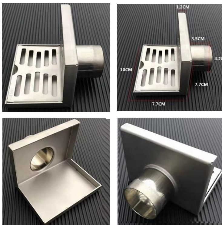
Kích thước Thoát sàn ngang S22
