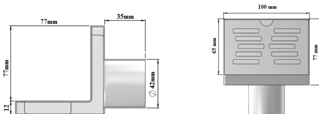
Kích thước Thoát sàn ngang S22
