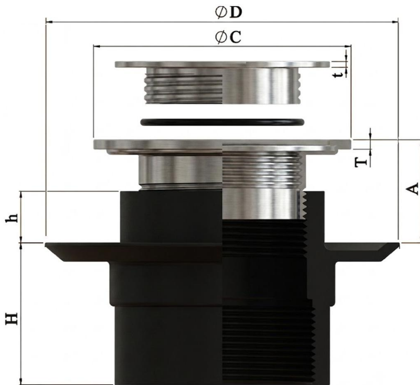
LỖ THOÁT REN TRONG/REN NGOÀI/TRƠN
